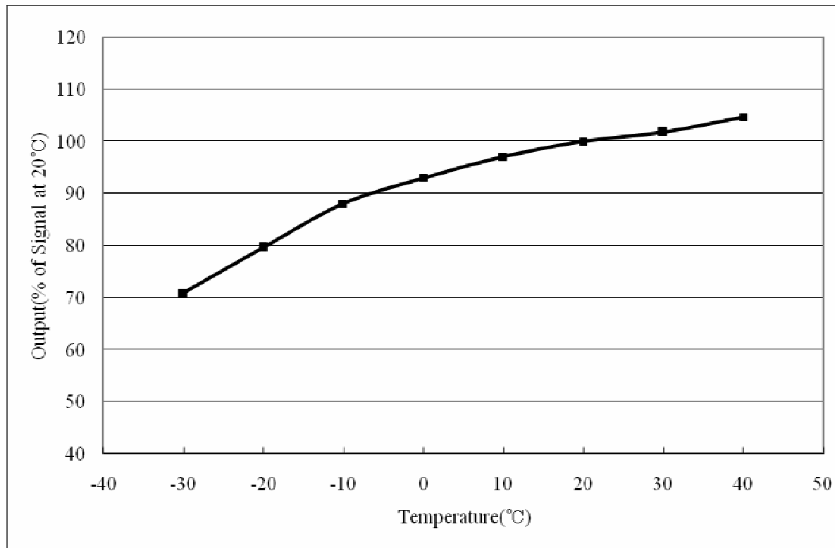
图3：NE-NH3的典型温度系数 (100 在20摄氏度时)
