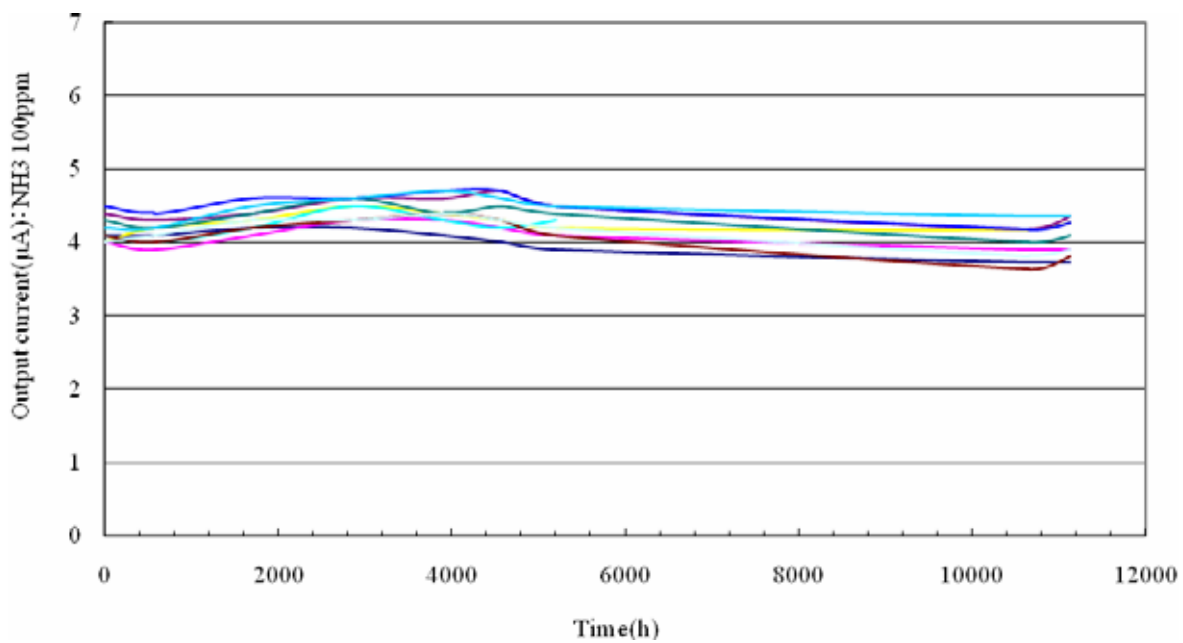
图5：NE-NH3常规环境下长期稳定性
