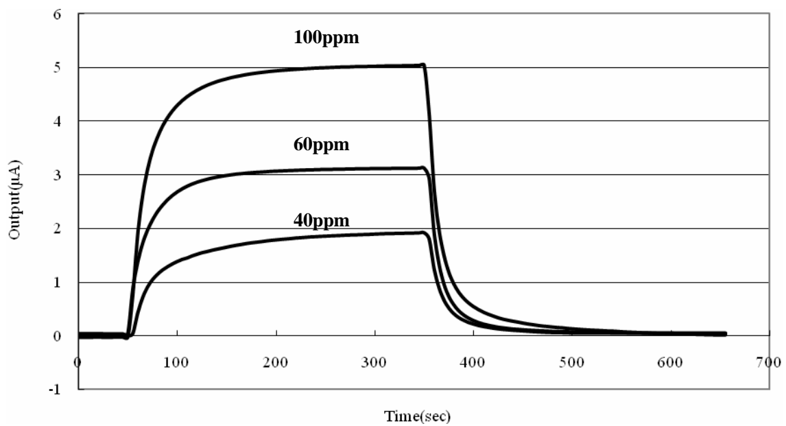
图4：反应和回复特性 (20 摄氏度时)
