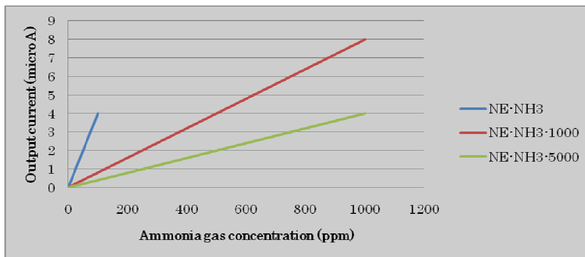
图2 : NE-NH3系列的气体灵敏度
