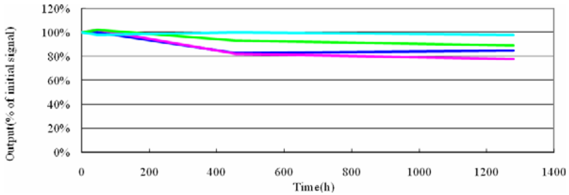
图8：高温高湿环境下的耐用性(50摄氏度 and 90%RH)
