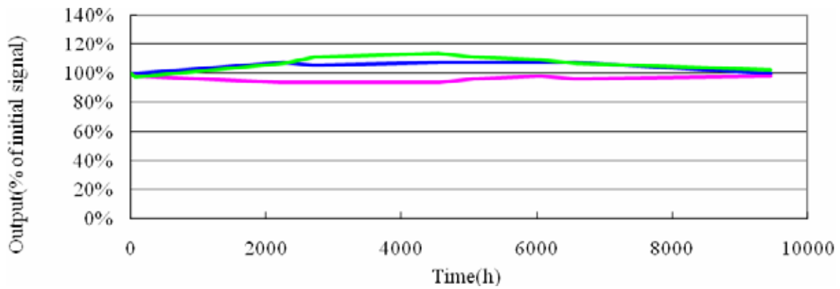
图9：低温环境下的耐用性 (零下20摄氏度)
