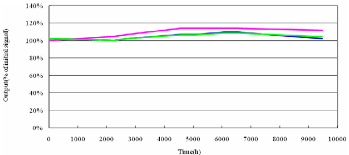
图7：高温干燥环境下的耐用性(50摄氏度)
