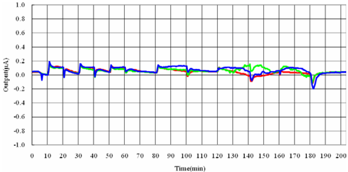
图6 :零点偏移变化的湿度变化依赖性
