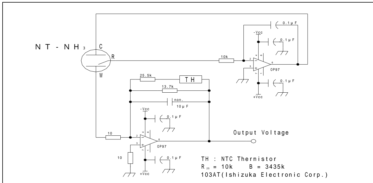
图10：检测评估电路图
