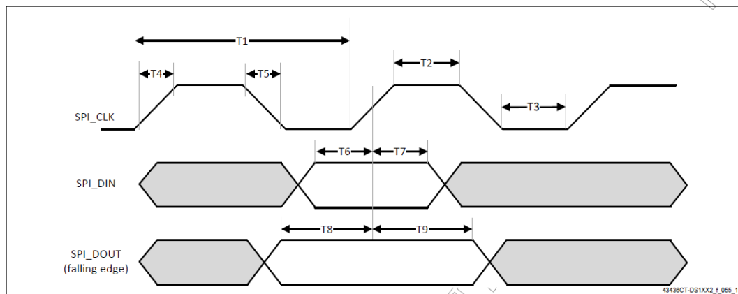
gSPI Timing Parameters
